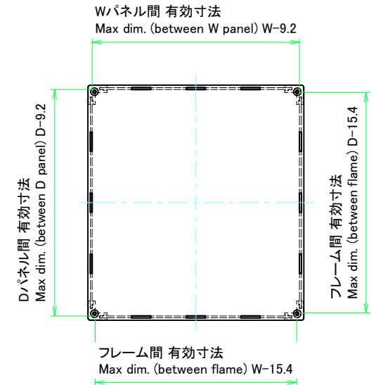
下カバー / Bottom cover
